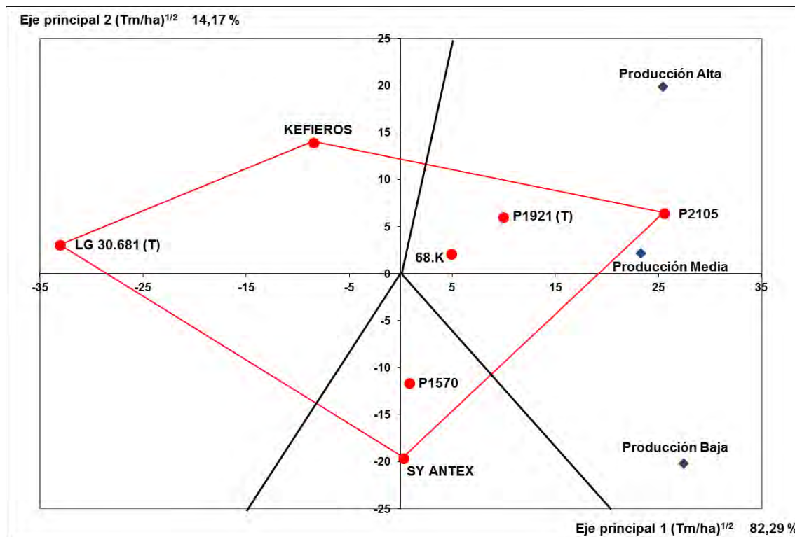
Figura 3.- Biplot G+GE realizado con los valores del PC1 y del PC2 obtenidos con los resultados productivos de las variedades de maíz convencionales de ciclo 700 ensayadas en el marco de GENVCE durante los años 2017 y 2018, en función de la productividad del ensayo.
